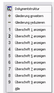
1 Dokumentstrukturbereich 2 Dokument
